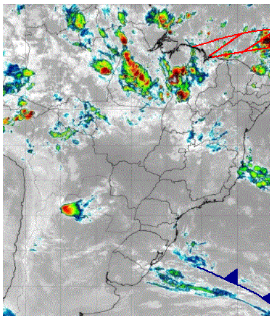
Figura 1. Sistemas sinóticos em superfície plotados sobre imagem de satélite da América do Sul. (Fonte: SIMGE, INMET e copyright 2018 GOES 16).
