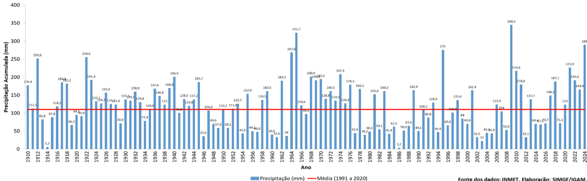
Figura 6: Série Histórica de Precipitação (mm) para o mês de outubro, na Estação Convencional de Belo Horizonte/INMET. Período: 1910 até 2024.
