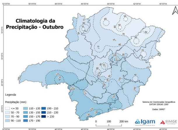
Figura 1: Distribuição espacial: (a) da Climatologia da precipitação mensal para outubro; (b) acumulado da precipitação em outubro de 2024; (c) Anomalia de precipitação em outubro de 2024.
