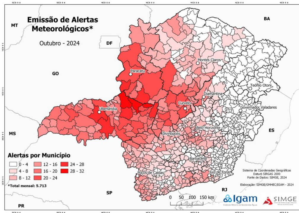
Figura 3: Distribuição espacial de Emissão de Alertas Meteorológicos no mês de outubro de 2024 em Minas Gerais.
