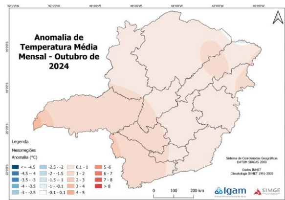
Figura 2: Distribuição espacial: (a) da Temperatura Mínima absoluta em outubro de 2024; (b) Temperatura Máxima absoluta em outubro de 2024; (c) Anomalia de temperatura média mensal em outubro de 2024.
