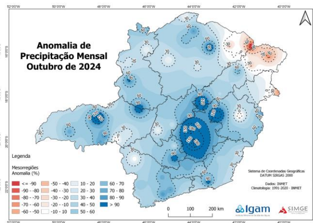
Figura 1: Distribuição espacial: (a) da Climatologia da precipitação mensal para outubro; (b) acumulado da precipitação em outubro de 2024; (c) Anomalia de precipitação em outubro de 2024.
