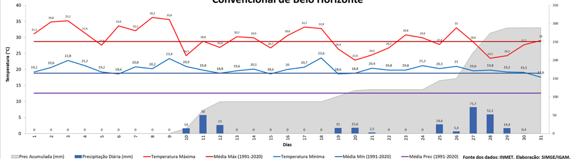
Figura 7: Precipitação Diária (mm), Temperatura Máxima e Mínima (°C) no mês de outubro de 2024 em Comparação com a Média Histórica (1991-2020), na Estação Convencional de Belo Horizonte/INMET.
