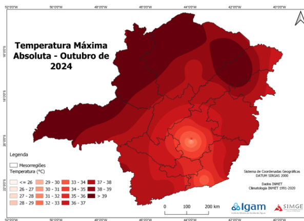
Figura 2: Distribuição espacial: (a) da Temperatura Mínima absoluta em outubro de 2024; (b) Temperatura Máxima absoluta em outubro de 2024; (c) Anomalia de temperatura média mensal em outubro de 2024.
