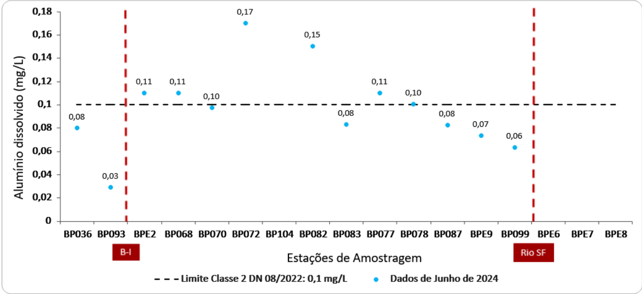
Figura 2 - Resultados de alumínio dissolvido para junho de 2024
