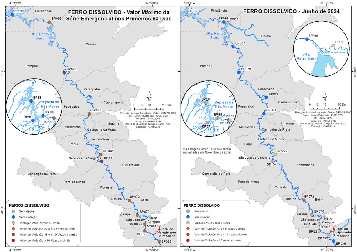
Figura 14 - Resultados dos valores máximos de ferro dissolvido para cada estação de monitoramento nos primeiros 60 dias após o rompimento da B-I e os resultados do mês de junho de 2024
