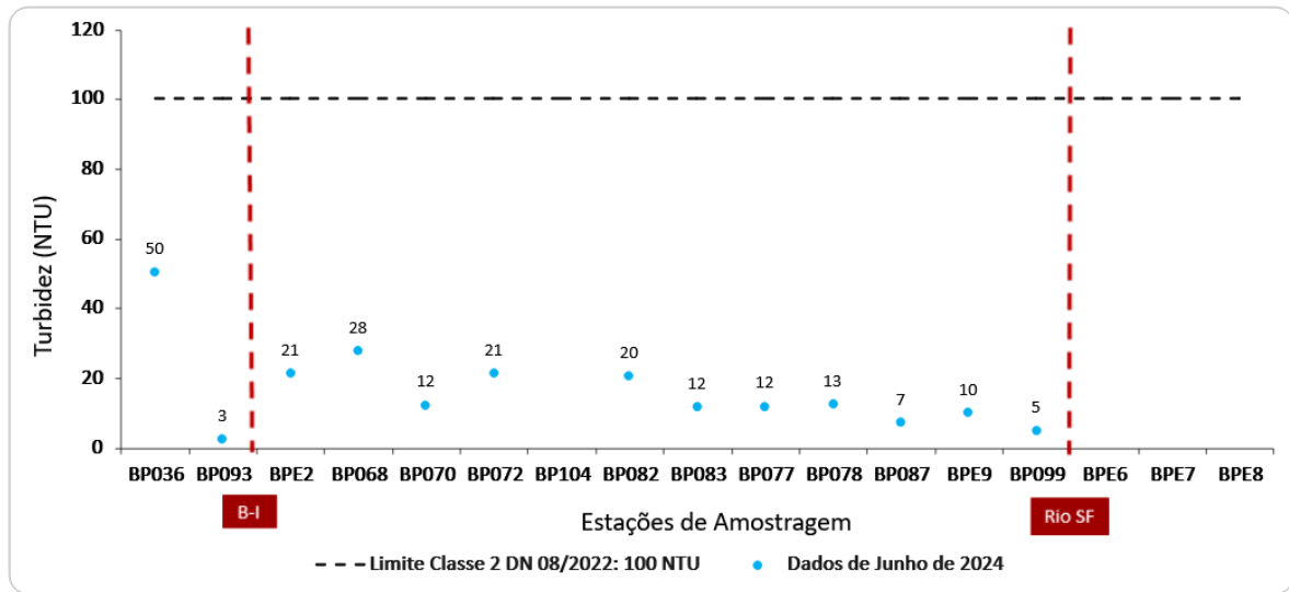
Figura 7 - Resultados de turbidez para junho de 2024
