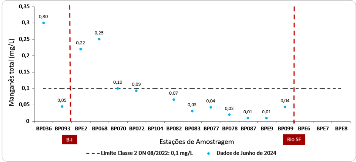
Figura 9 - Resultados de manganês total para junho de 2024
