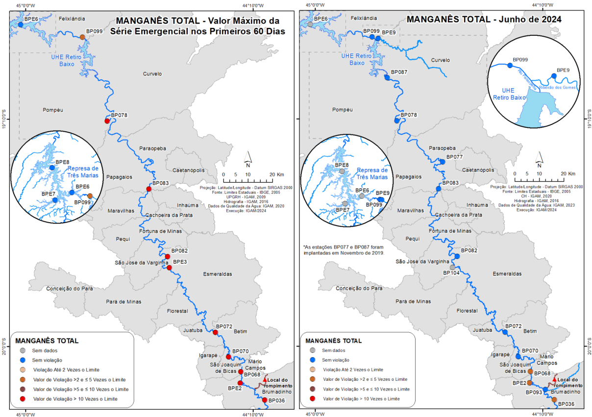
Figura 10 - Resultados de manganês total para cada estação de monitoramento nos primeiros 60 dias após o rompimento da B-I e os resultados do mês de junho de 2024
