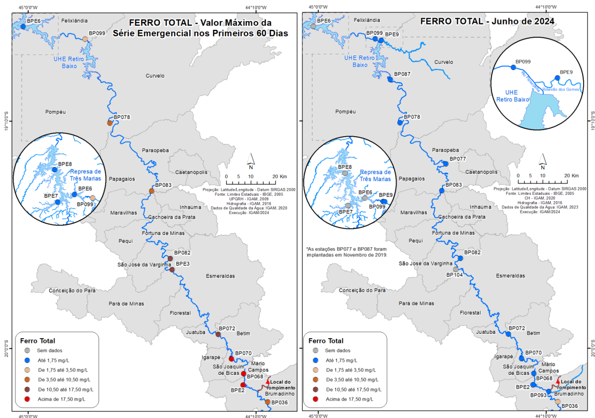
Figura 12 - Resultados dos valores máximos de ferro total para cada estação de monitoramento nos primeiros 60 dias após o rompimento da B-I e os resultados do mês de junho de 2024
