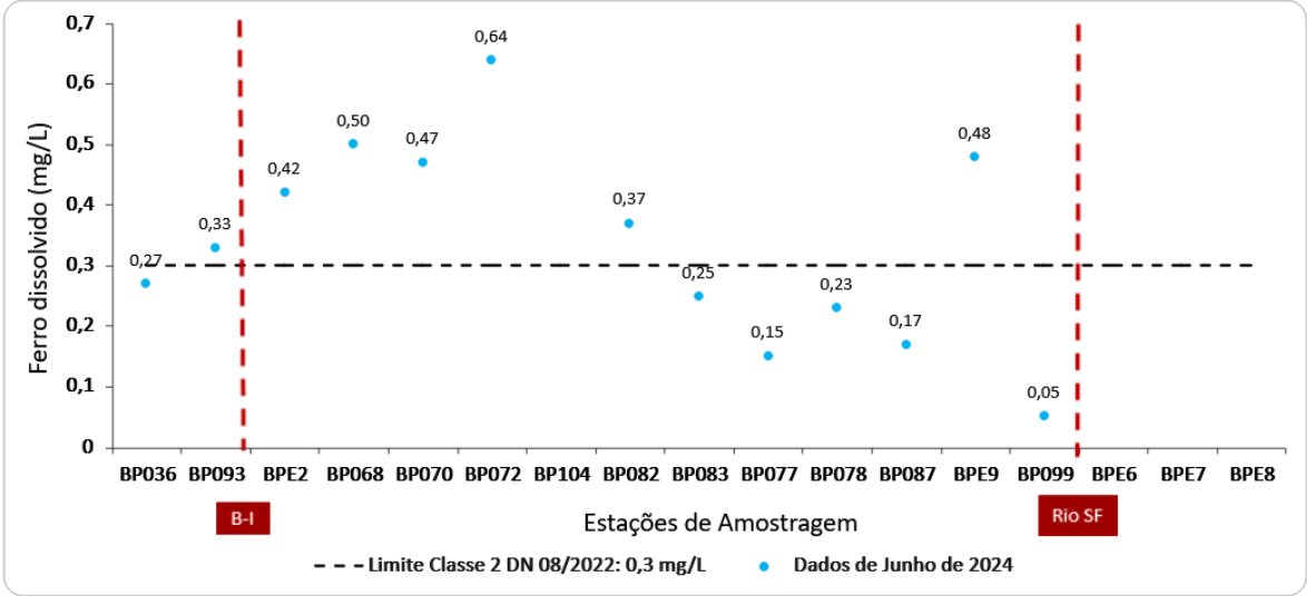
Figura 13 - Resultados de ferro dissolvido para junho de 2024
