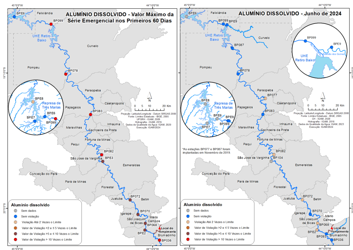
Figura 3 - Resultados dos valores máximos de alumínio dissolvido para cada estação de monitoramento nos primeiros 60 dias após o rompimento da B-I e os resultados do mês de junho de 2024
