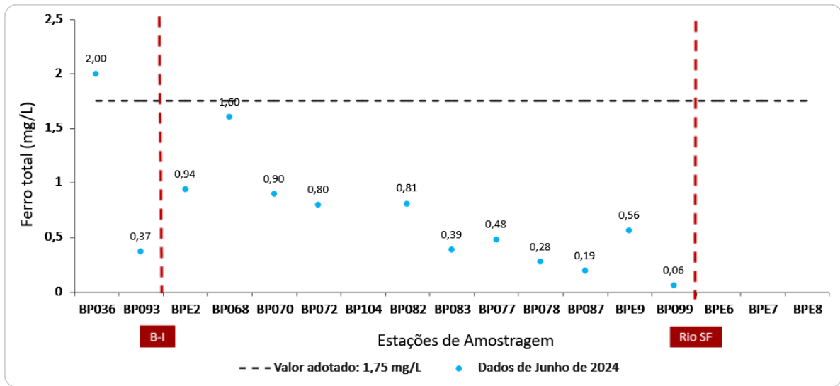
Figura 11 - Resultados de ferro total para junho de 2024
