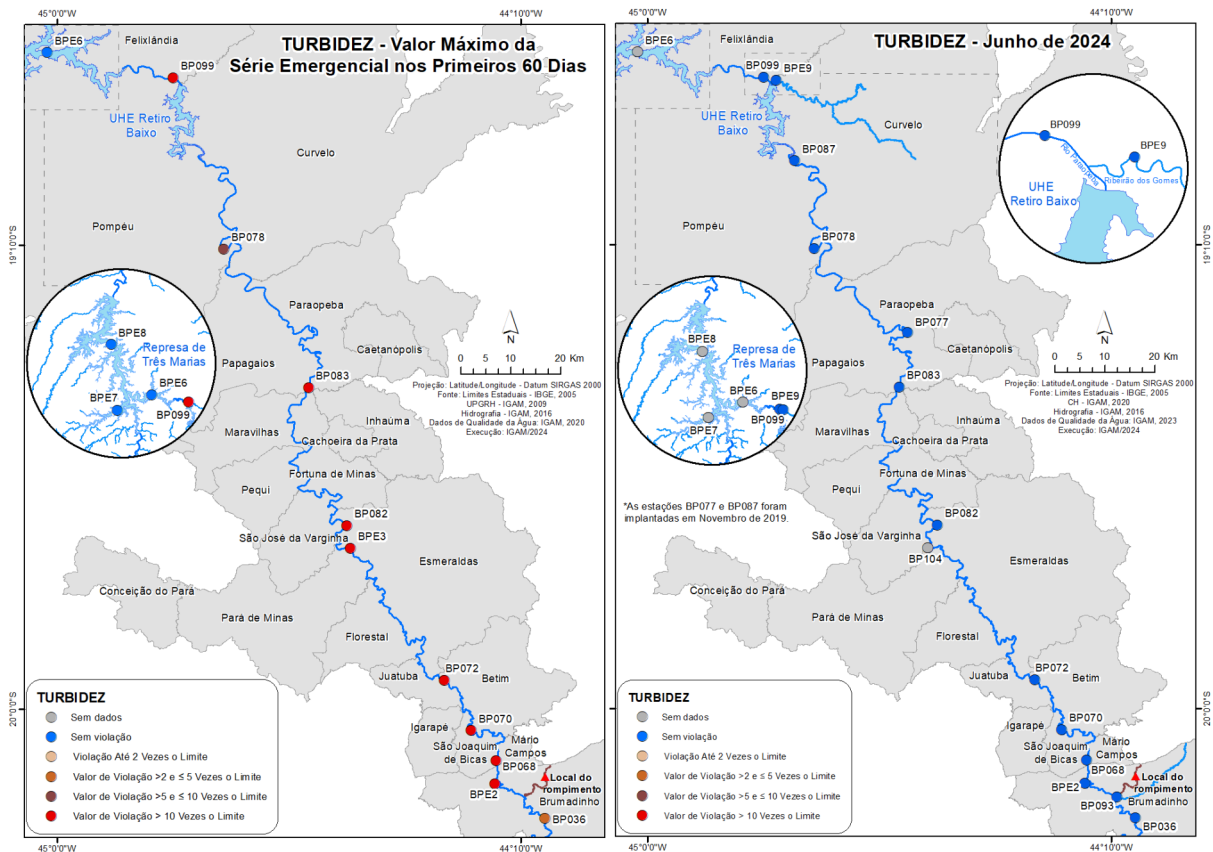
Figura 8 - Resultados dos valores máximos de turbidez para cada estação de monitoramento nos primeiros 60 dias após o rompimento da B-I e os resultados do mês de junho de 2024
