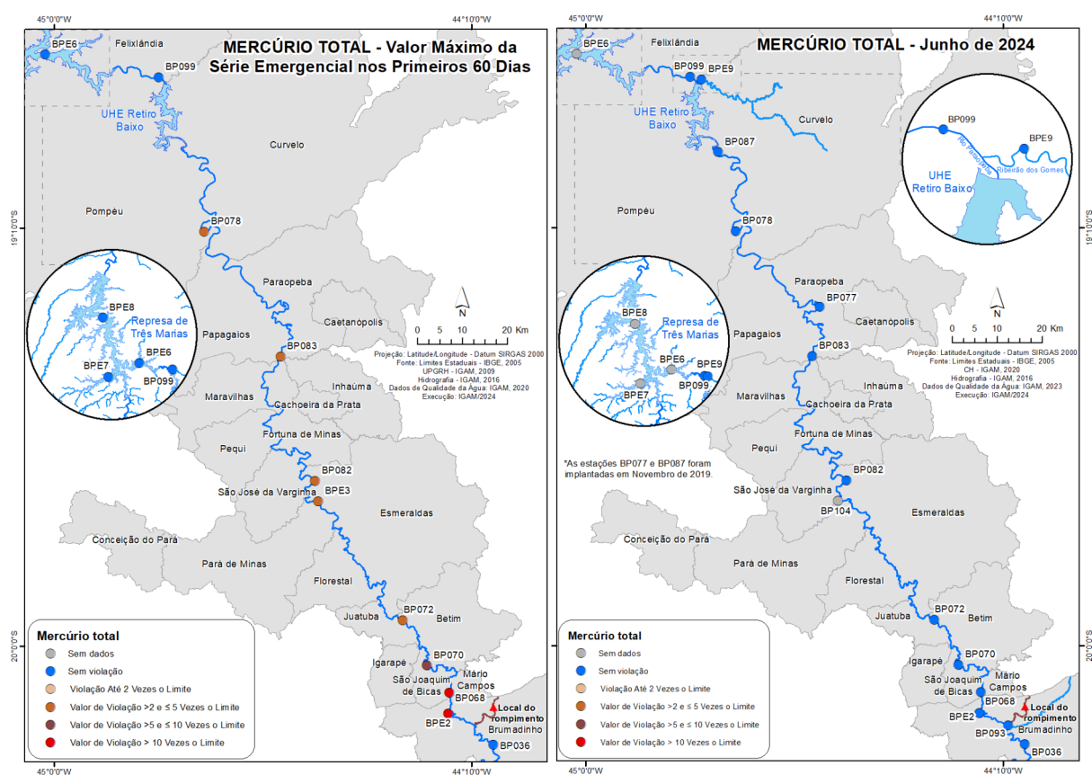
Figura 6 - Resultados dos valores máximos de mercúrio total para cada estação de monitoramento nos primeiros 60 dias após o rompimento da B-I e os resultados do mês de junho de 2024
