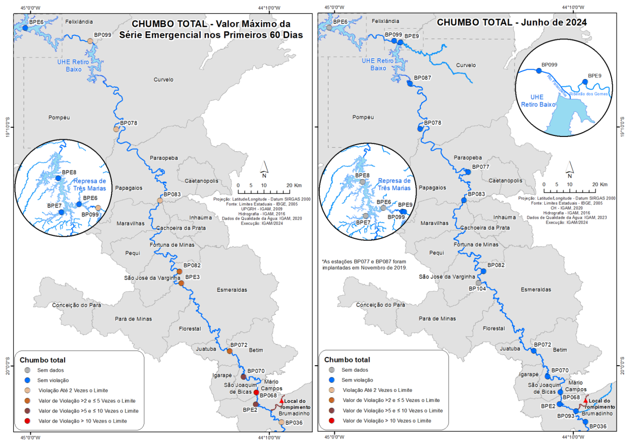
Figura 5 - Resultados dos valores máximos de chumbo total para cada estação de monitoramento nos primeiros 60 dias após o rompimento da B-I e os resultados do mês de junho de 2024
