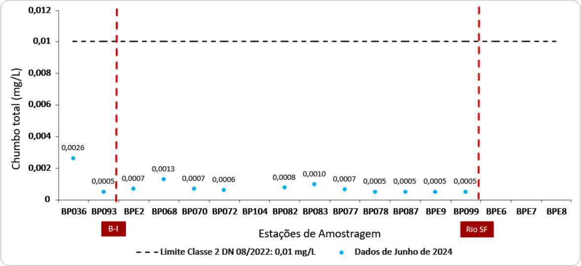
Figura 4 - Resultados de chumbo total para junho de 2024
