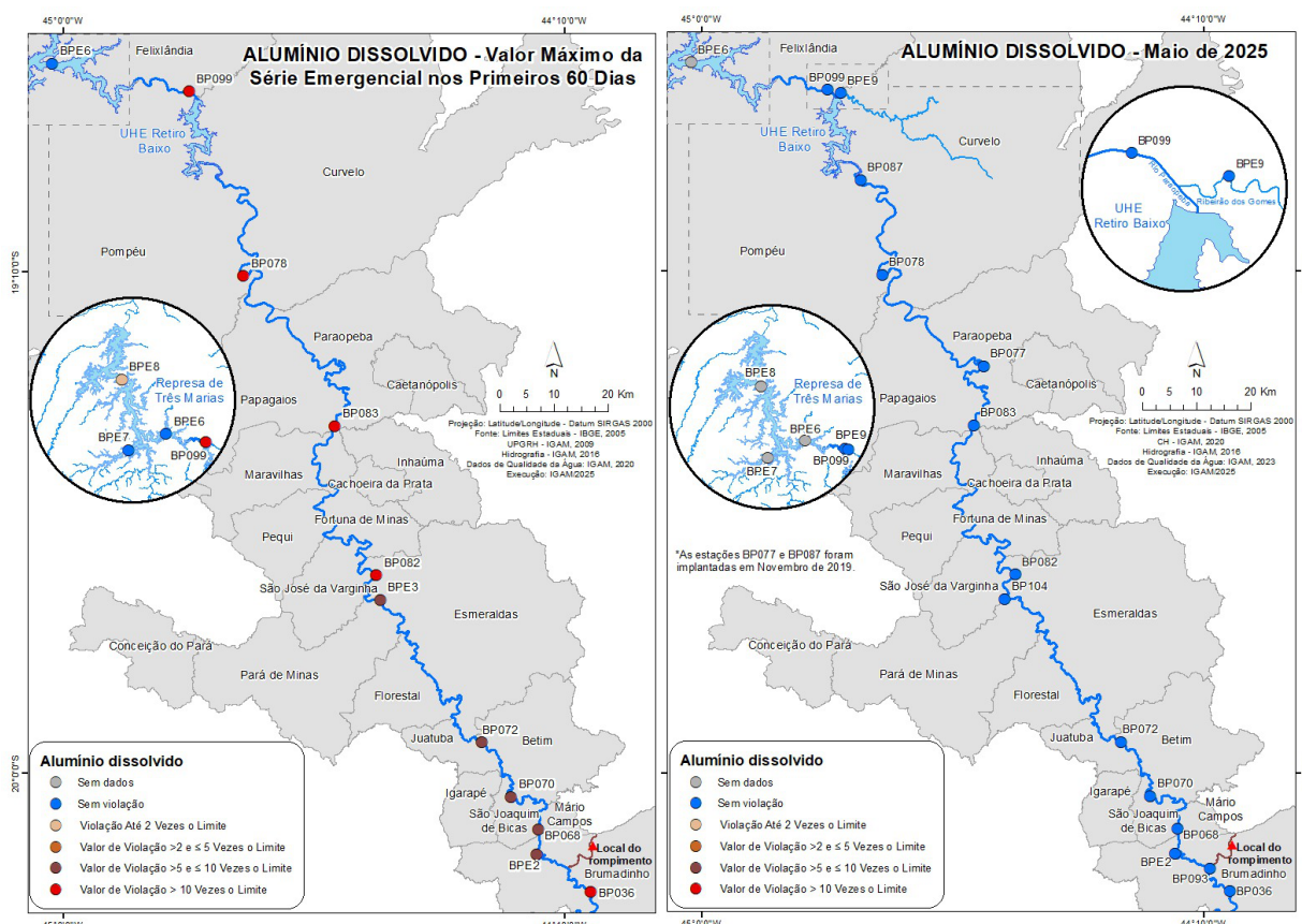
Figura 3 - Resultados dos valores máximos de alumínio dissolvido para cada estação de monitoramento nos primeiros 60 dias após o rompimento da B-I e os resultados do mês de maio de 2025
