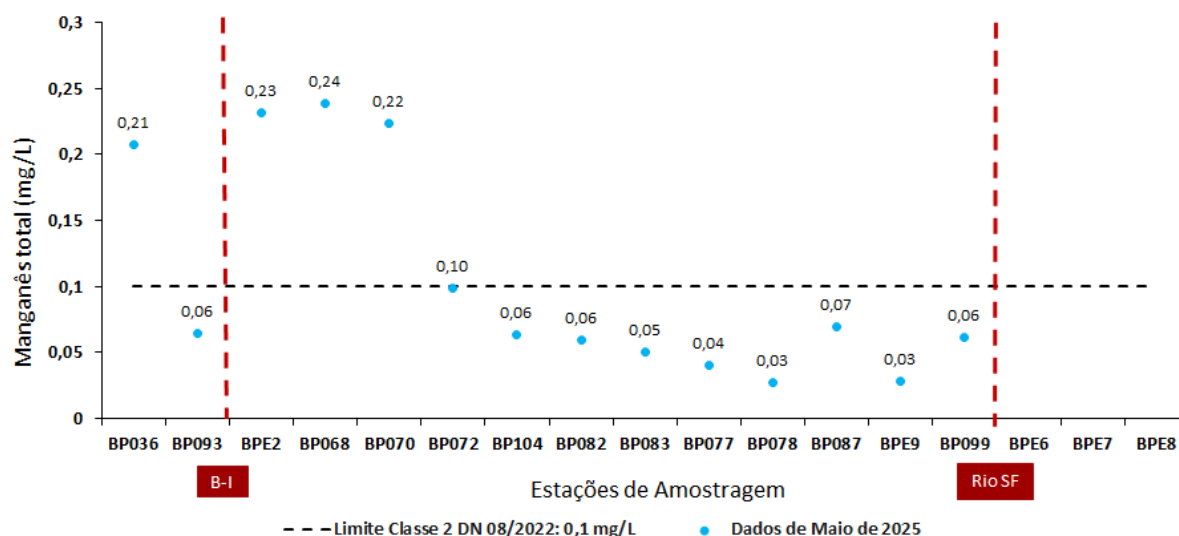
Figura 9 - Resultados de manganês total maio de 2025
