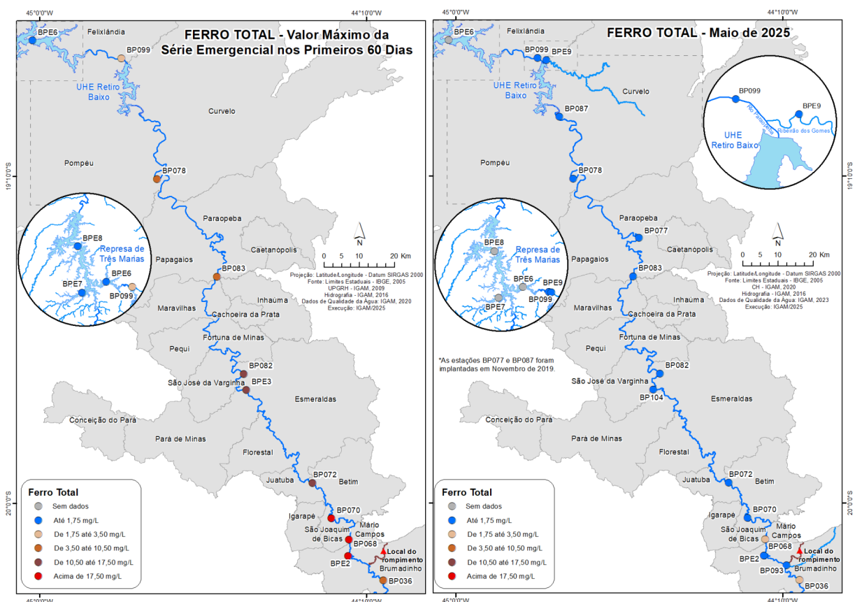
Figura 12 - Resultados dos valores máximos de ferro total para cada estação de monitoramento nos primeiros 60 dias após o rompimento da B-I e os resultados do mês de maio de 2025
