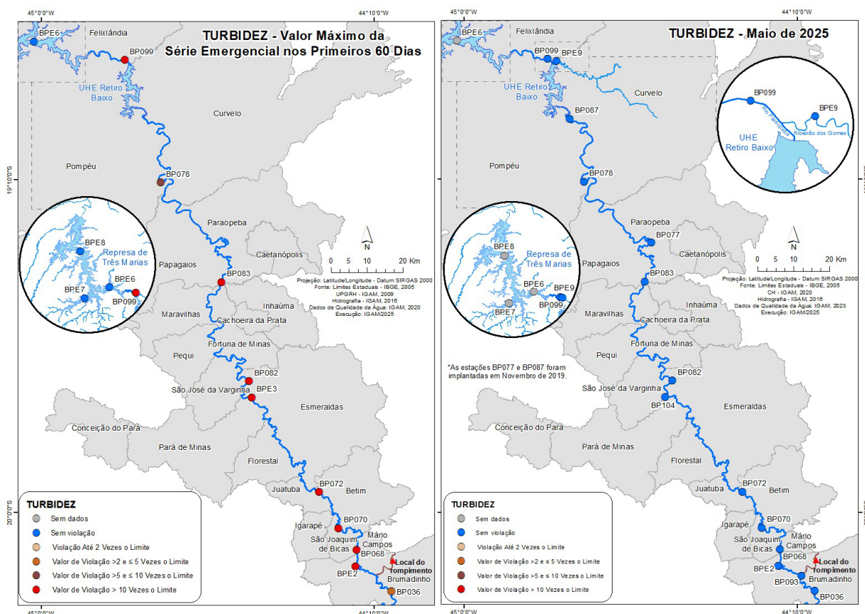
Figura 8 - Resultados dos valores máximos de turbidez para cada estação de monitoramento nos primeiros 60 dias após o rompimento da B-I e os resultados do mês de maio de 2025
