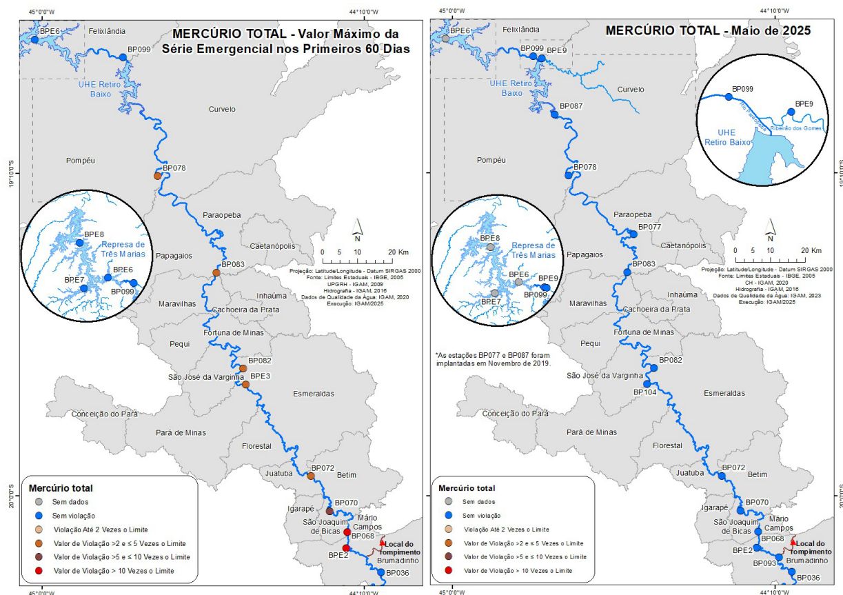
Figura 6 - Resultados dos valores máximos de mercúrio total para cada estação de monitoramento nos primeiros 60 dias após o rompimento da B-I e os resultados do mês de maio de 2025
