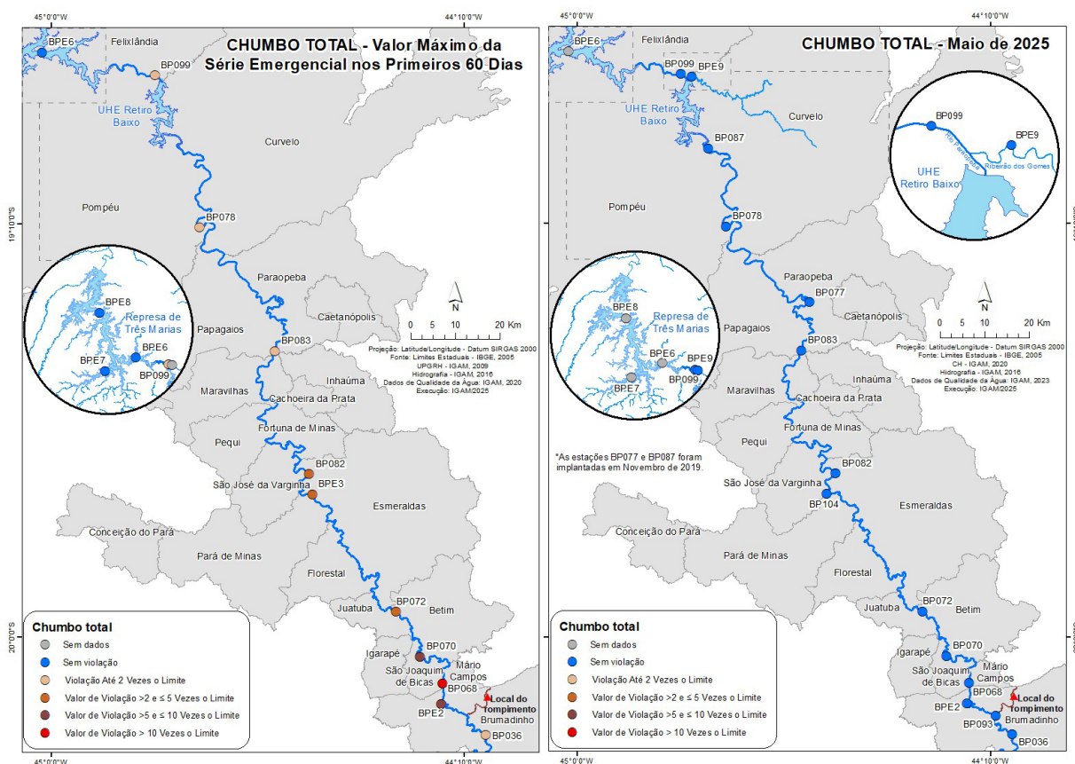
Figura 5 - Resultados dos valores máximos de chumbo total para cada estação de monitoramento nos primeiros 60 dias após o rompimento da B-I e os resultados do mês de maio de 2025
