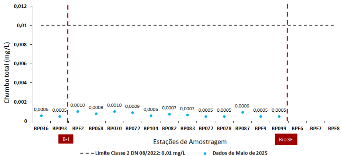
Figura 4 - Resultados de chumbo total para maio de 2025
