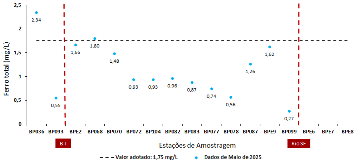
Figura 11 - Resultados de ferro total para maio de 2025
