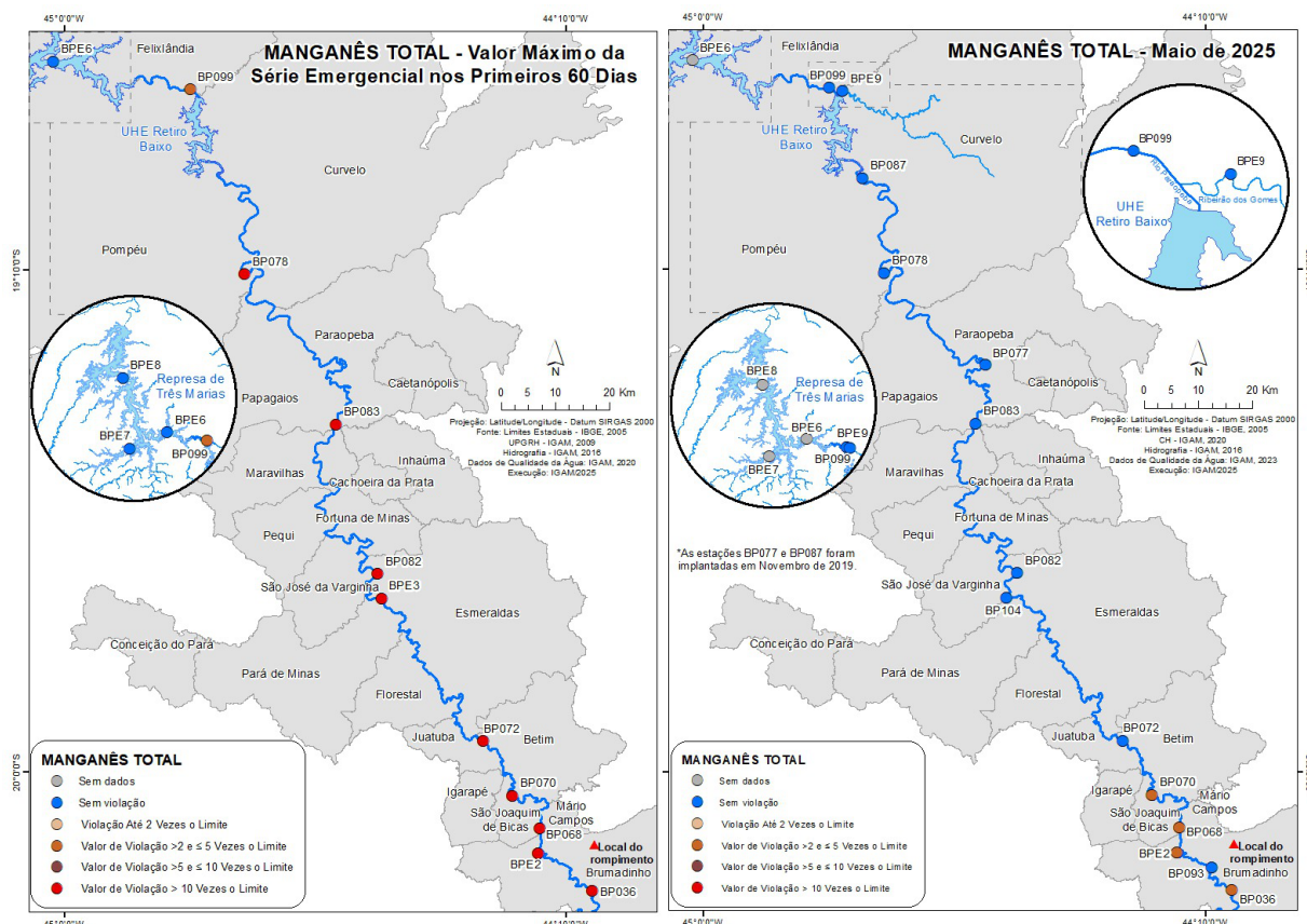
Figura 10 - Resultados de manganês total para cada estação de monitoramento nos primeiros 60 dias após o rompimento da B-I e os resultados do mês de maio de 2025
