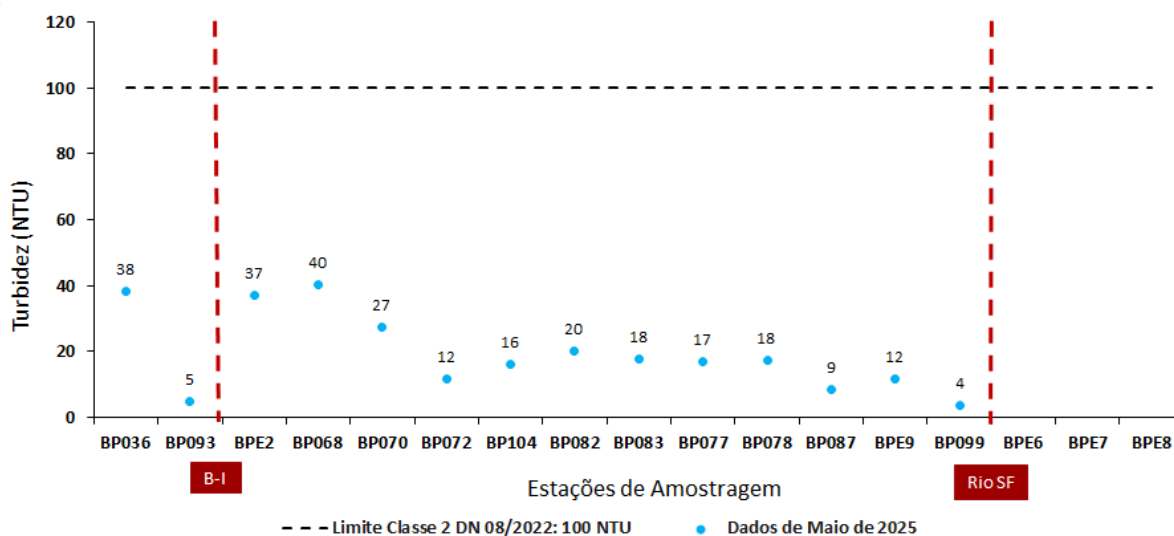
Figura 7 - Resultados de turbidez para maio de 2025
