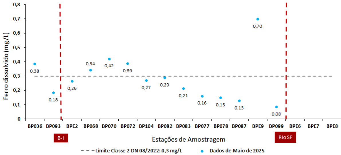
Figura 13 - Resultados de ferro dissolvido para maio de 2025
