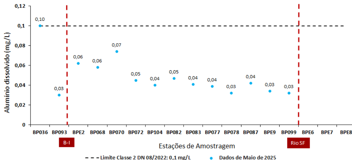
Figura 2 - Resultados de alumínio dissolvido para maio de 2025
