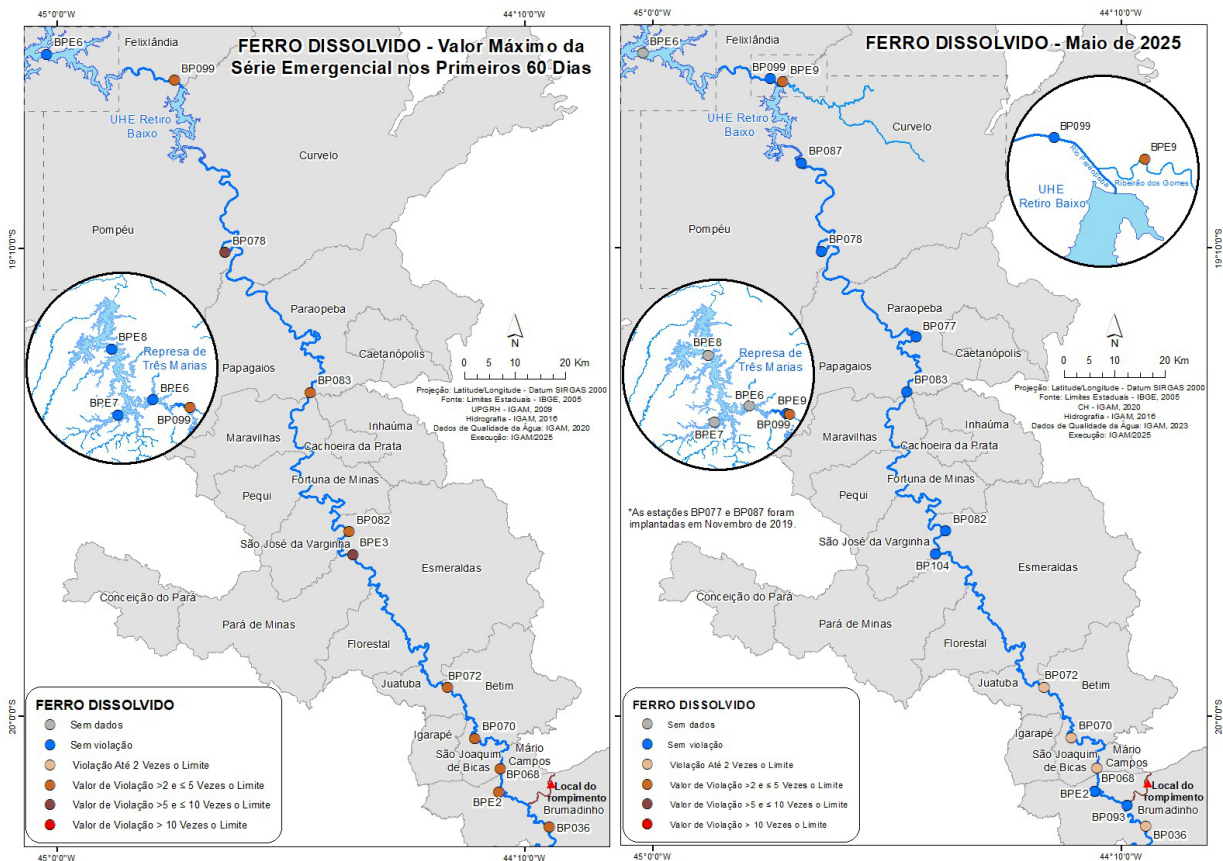
Figura 14 - Resultados dos valores máximos de ferro dissolvido para cada estação de monitoramento nos primeiros 60 dias após o rompimento da B-I e os resultados do mês de maio de 2025
